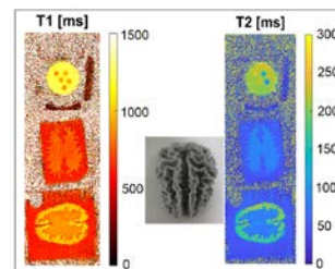
Misura dei tempi di rilassamento T1 e T2 su un phantom antropomorfo realizzato all'INRiM, per la caratterizzazione di tecniche di diagnostica MRI di tipo quantitativo.
