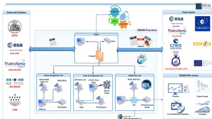
Architettura dell'infrastruttura Galileo dell'INRiM.
