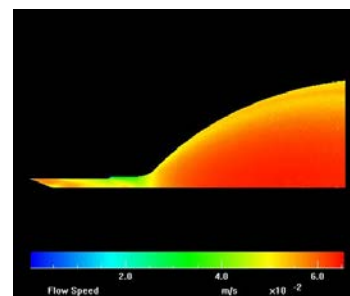
Mappa di velocità del flusso (simulato) in ugello per micropropulsore.
