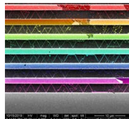
Architetture di self-assembly direzionato per nanosfere di polistirene.
