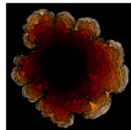
Espansione di una bolla magnetica di circa 100 nm in presenza di un campo magnetico perpendicolare con una dinamica detta di 'creep' su un film sottile di FeCoB/MgO di 1nm di spessore.
