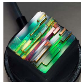
Filtro V(\lambda) a mosaico.
